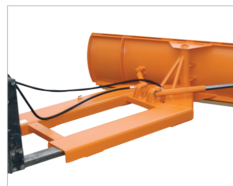
Hydraulische Schildverstellung
